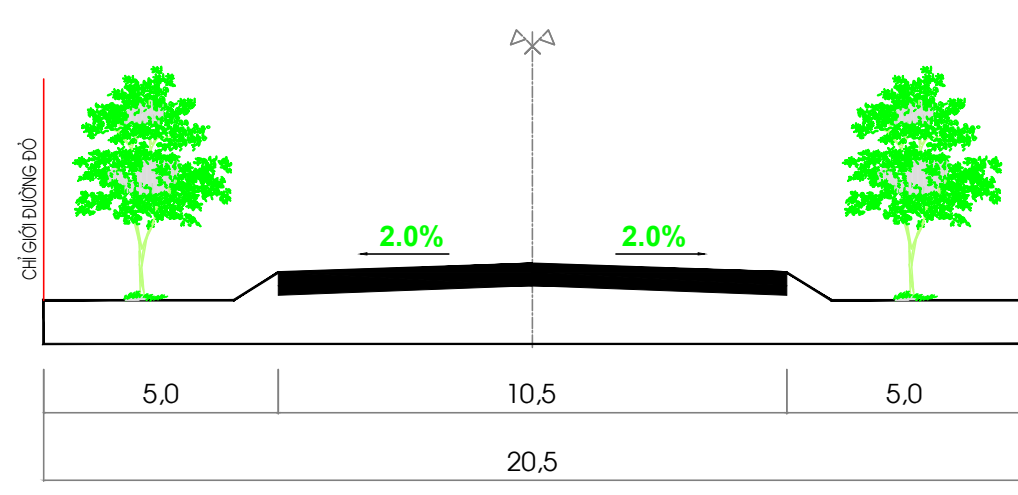
MẶT CẮT 2 - 2 ĐƯỜNG SANG TT TỨ KỲ
