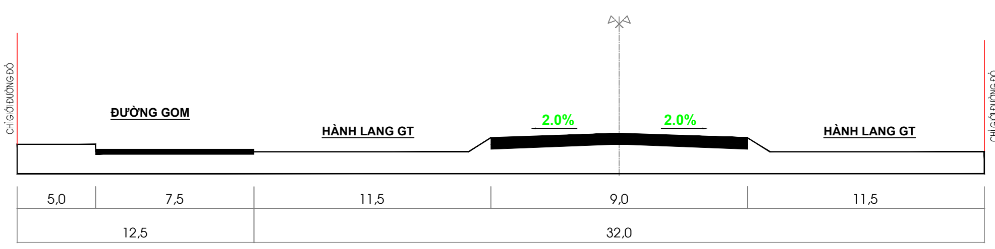
MẶT CẮT 1' - 1' ĐƯỜNG HUYỆN (ĐOẠN QUA ĐẤT THƯƠNG MẠI DỊCH VỤ, KHU DÂN CƯ QUY HOẠCH MỚI)
