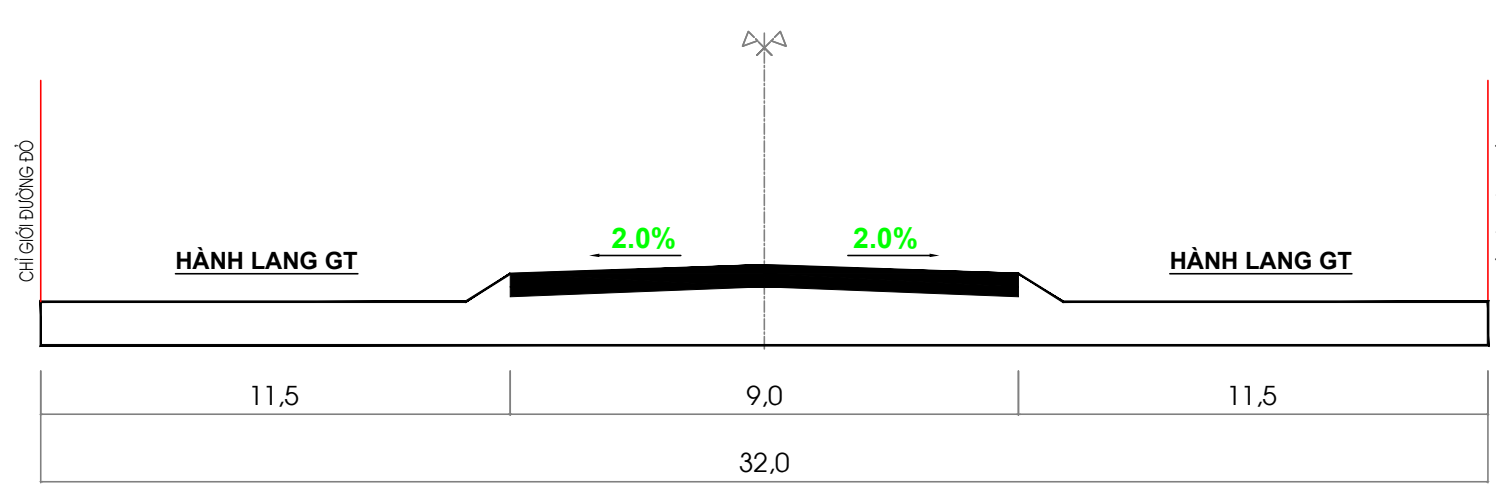
MẶT CẮT 1 - 1 ĐƯỜNG HUYỆN (ĐOẠN QUA KHU DÂN CƯ HIỆN TRẠNG)
