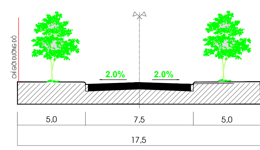
MẶT CẮT 3 - 3 ĐƯỜNG XÃ
