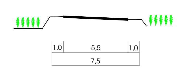
MẶT CẮT 5 - 5 ĐƯỜNG NGÕ XOM
