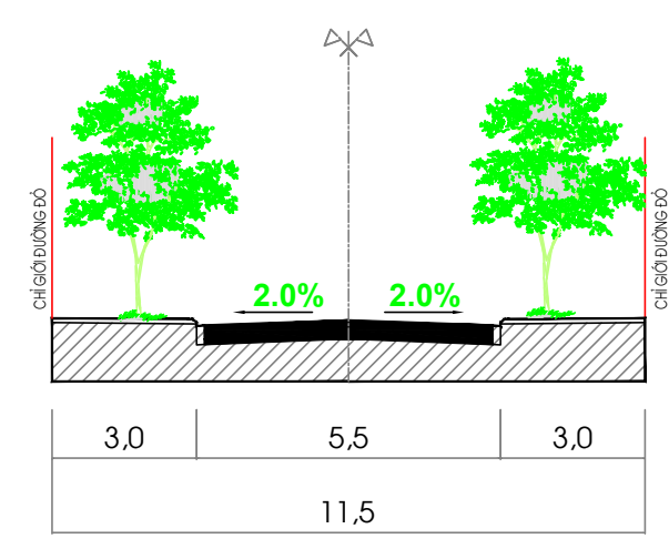
MẶT CẮT 4 - 4 ĐƯỜNG THÔN
