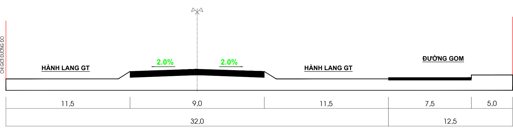
MẶT CẮT 1'' - 1'' ĐƯỜNG HUYỆN (ĐOẠN QUA ĐẤT CÔNG NGHIỆP)
