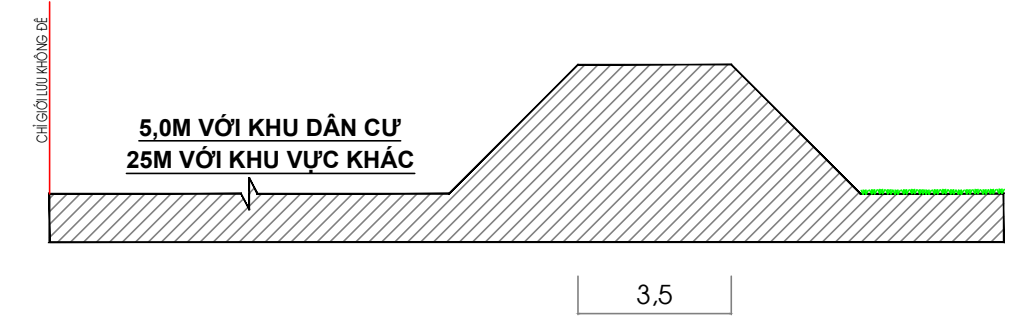
MẶT CẮT 6 - 6 ĐƯỜNG ĐÈ
